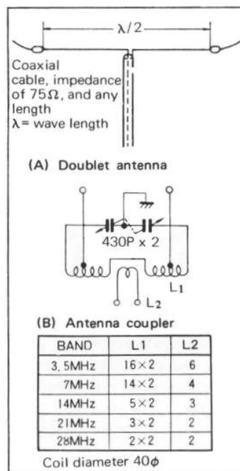
Fig. 13. ANT Coupler
